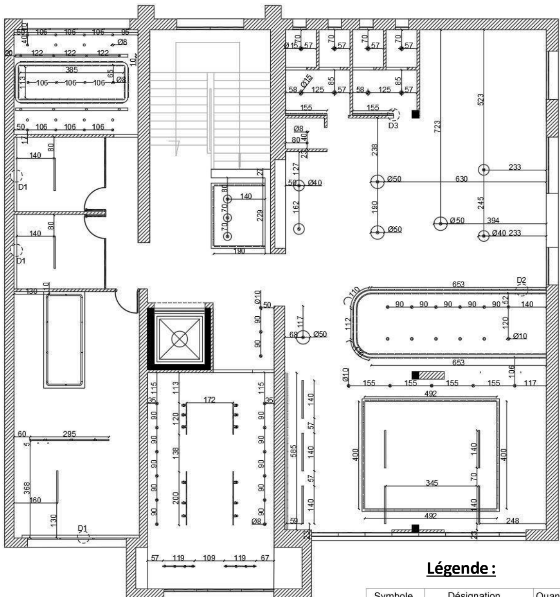
Plan faux plafond éclairage
