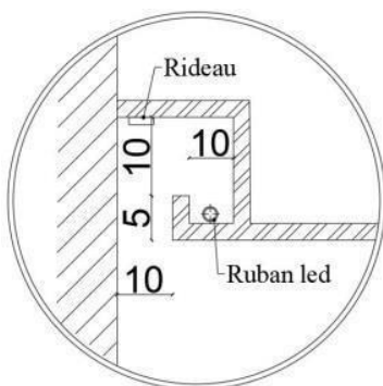
Détail 1:Cache rideau / Cache lumière
