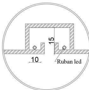
Détail 3: Cache lumière
